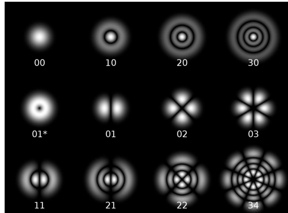
Laguerre-Gauss
