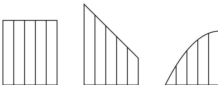
Slika 7.1: D'Oresmeov prikaz latituda u ovisnosti o longitudama.
