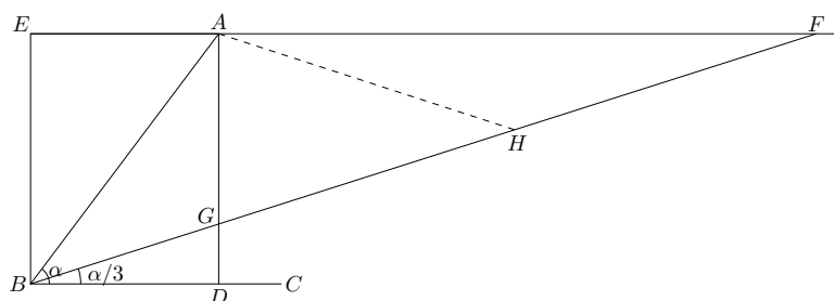
Slika 4.10: Hipokratova trisekcija kuta.
