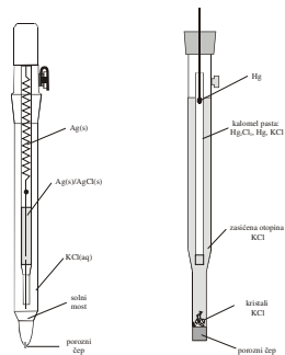
Referentne elektrode: srebro/srebrov klorid; kalomelova elektroda.
