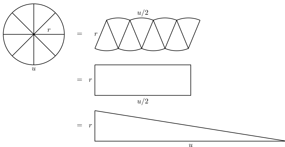
Slika 4.30: Arhimedov teorem o krugu
