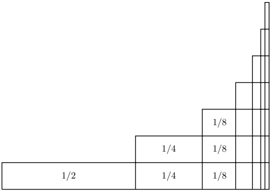
Slika 7.2: Ilustracija dokaza da je \sum_n \frac{n}{2^n} = 2 .
