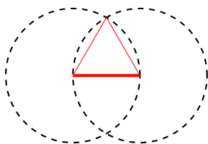
Slika 4.16: Konstrukcija jednakostraničnog trokuta u EEI1
