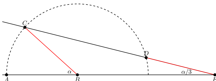
Slika 4.34: Arhimedova trisekcija kuta
