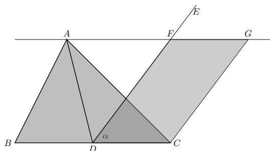
Slika 4.17: Konstrukcija paralelograma zadanog kuta jednakog zadanom trokutu (EEI42).
