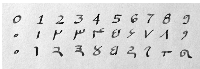
Slika 6.1: Usporedba ranih arapskih znamenki (drugi red) i nagari-znamenki (treći red).
