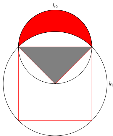
Slika 4.8: Prvi Hipokratov mjesec.
