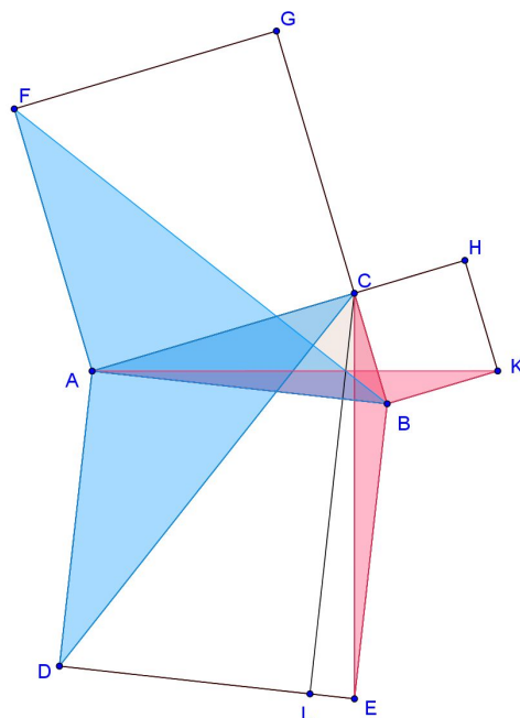
Slika 4.1: Ilustracija uz Euklidov dokaz nužnosti u Pitagorinom poučku.
