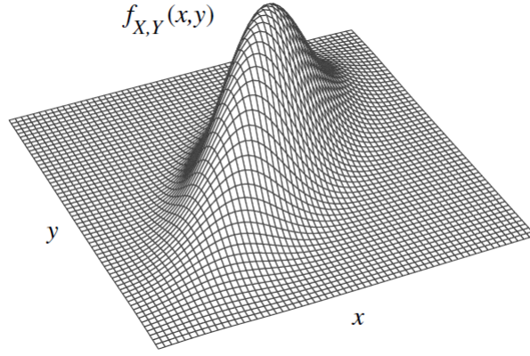
SLIKA 8. Primjer zajedničke gustoće – za svaki A \subseteq \mathbb{R}^2 , \mathbb{P}((X,Y) \in A) je volumen skupa \{(x,y,z) \in \mathbb{R}^3 : (x,y) \in A, 0 \leq z \leq f(x,y)\} . Preuzeto iz [BH19].
