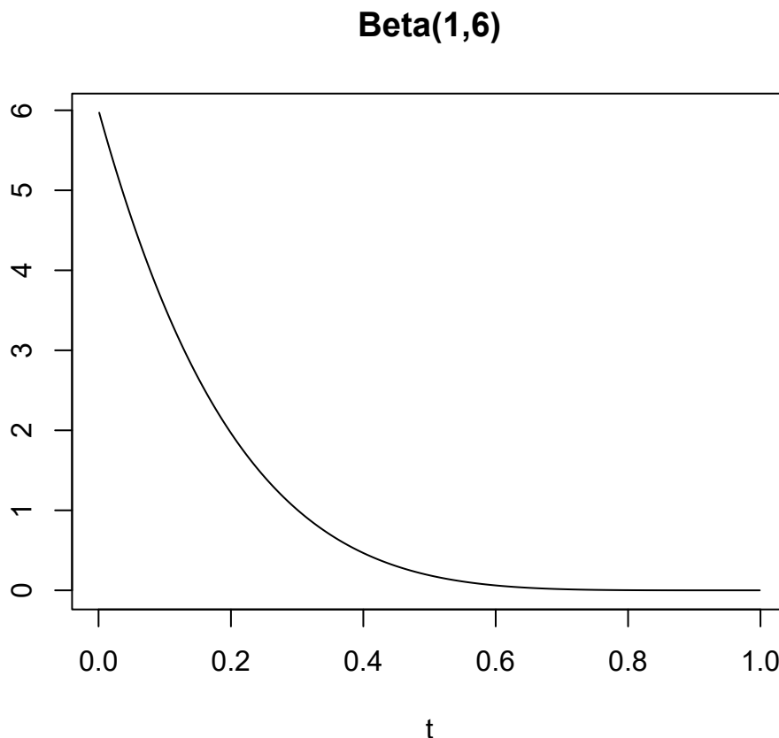
SLIKA 12. Aposteriorna razdioba za P u Primjeru 7.16, i to u slučaju uniformne apriorne razdiobe, n = 5 i N_n = 0 . Dakle, u Bayesovskom pristupu dobivamo cijelu razdiobu za parametra koji procjenjujemo!
